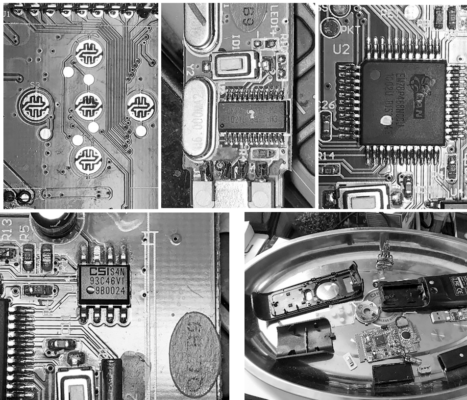
Hình 8: Chụp hình thực tế từ board mạch Laser Presenter Lexma Model: MP8
