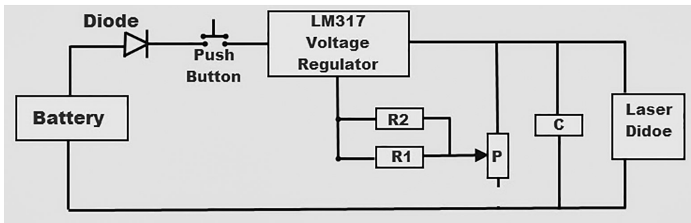
Hình 4: Mạch điều khiển con trở laser.
